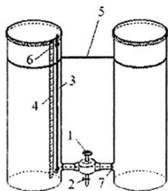
Hình B.1 - Thiết bị cấp nước - các thùng đo định chuẩn
